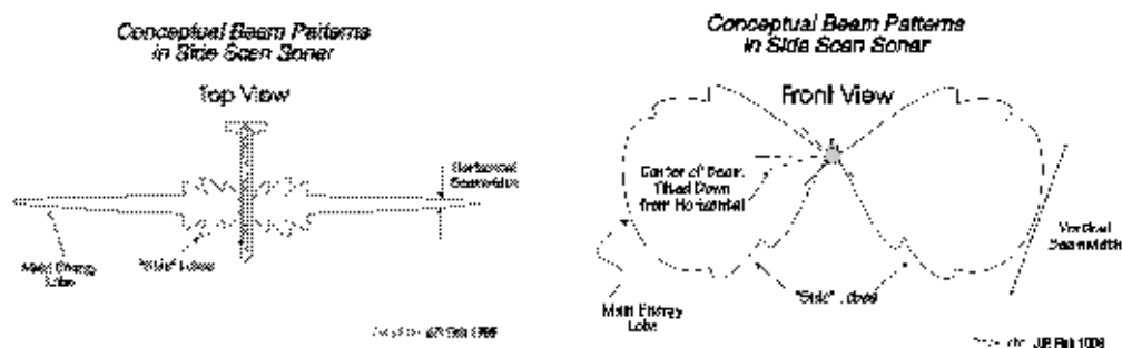
Figuur 2, Sidescan sonar bundels
