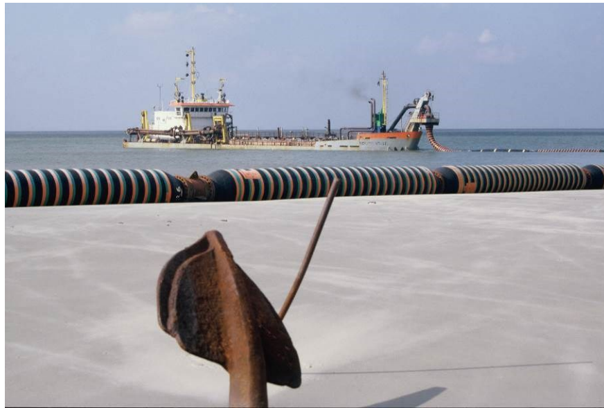
Foto 4.14. Zandsuppletie. (Foto RWS)
