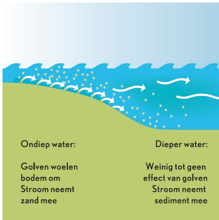
Figuur 2.1. Werking van golven en stroom (Lit. 67).
