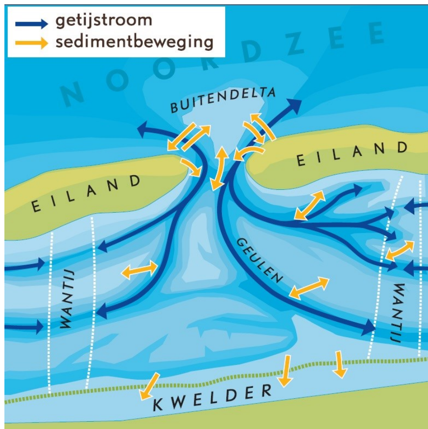
Figuur 2.2. Getijstroom en sedimentbeweging rond de waddeneilanden (Lit. 51)
