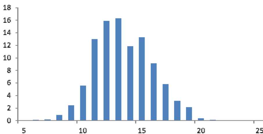
Figuur 28 Lengte klassen verdeling in mm van de witte dunschaal in % van het totaal aantal gemeten dieren in 2011
