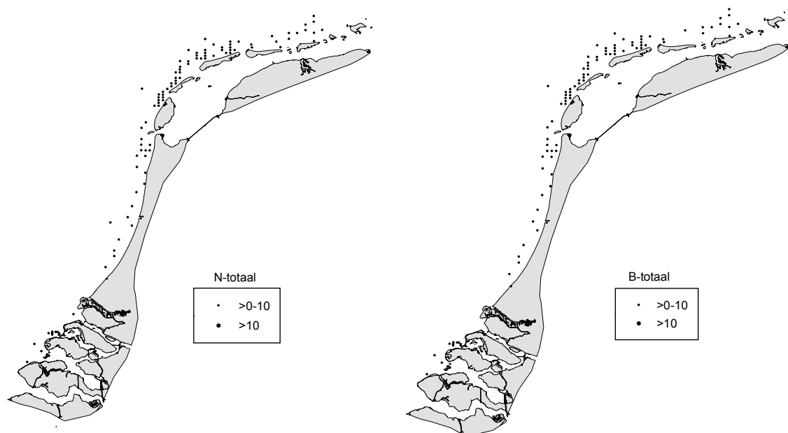
Figuur 31 Berekende dichtheid (aantal \text{m}^{-2} ) per locatie (links) en biomassa (rechts) van de tere platschelp in 2011
