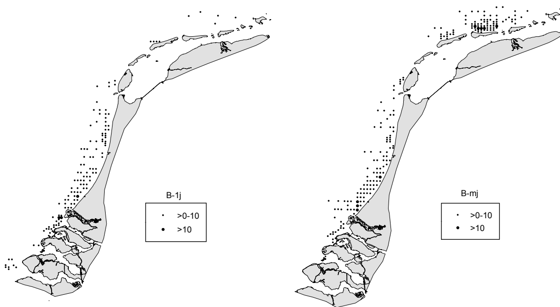
Figuur 7 Berekende biomassa (gram versgewicht \text{m}^{-2} ) per locatie van meerjarige (rechts) en 1-jarige dieren (links) in 2011.
