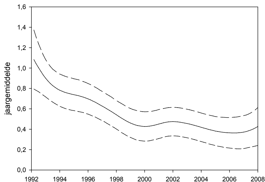
Figuur 3.4.3. Trend en 95% betrouwbaarheidsinterval van de Zilvermeeuw op het Nederlands Continentaal Plat (NCP) in 1992-2008. Trend with 95% confidence limits of Herring Gull on the Dutch Continental Shelf in 1992-2008.
