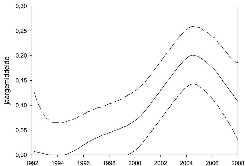
Figuur 3.9.3. Trend en 95% betrouwbaarheidsinterval van de Bruinvis op het Nederlands Continentaal Plat (NCP) in 1992-2008. Trend with 95% confidence limits of Harbour Porpoise on the Dutch Continental Shelf in 1992-2008.
