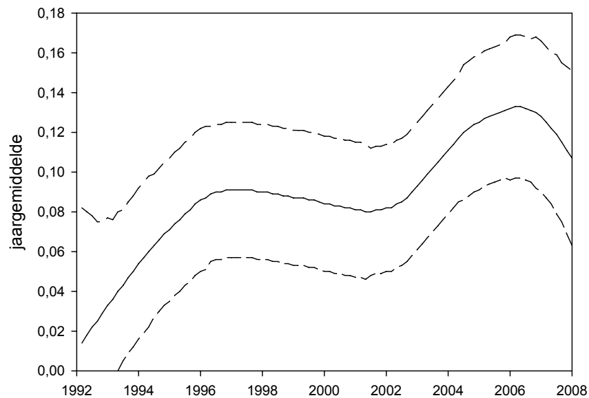
Figuur 3.6.3. Trend en 95% betrouwbaarheidsinterval van de Grote Stern op het Nederlands Continentaal Plat (NCP) in 1992-2008. Trend with 95% confidence limits of Sandwich Tern on the Dutch Continental Shelf in 1992-2008.
