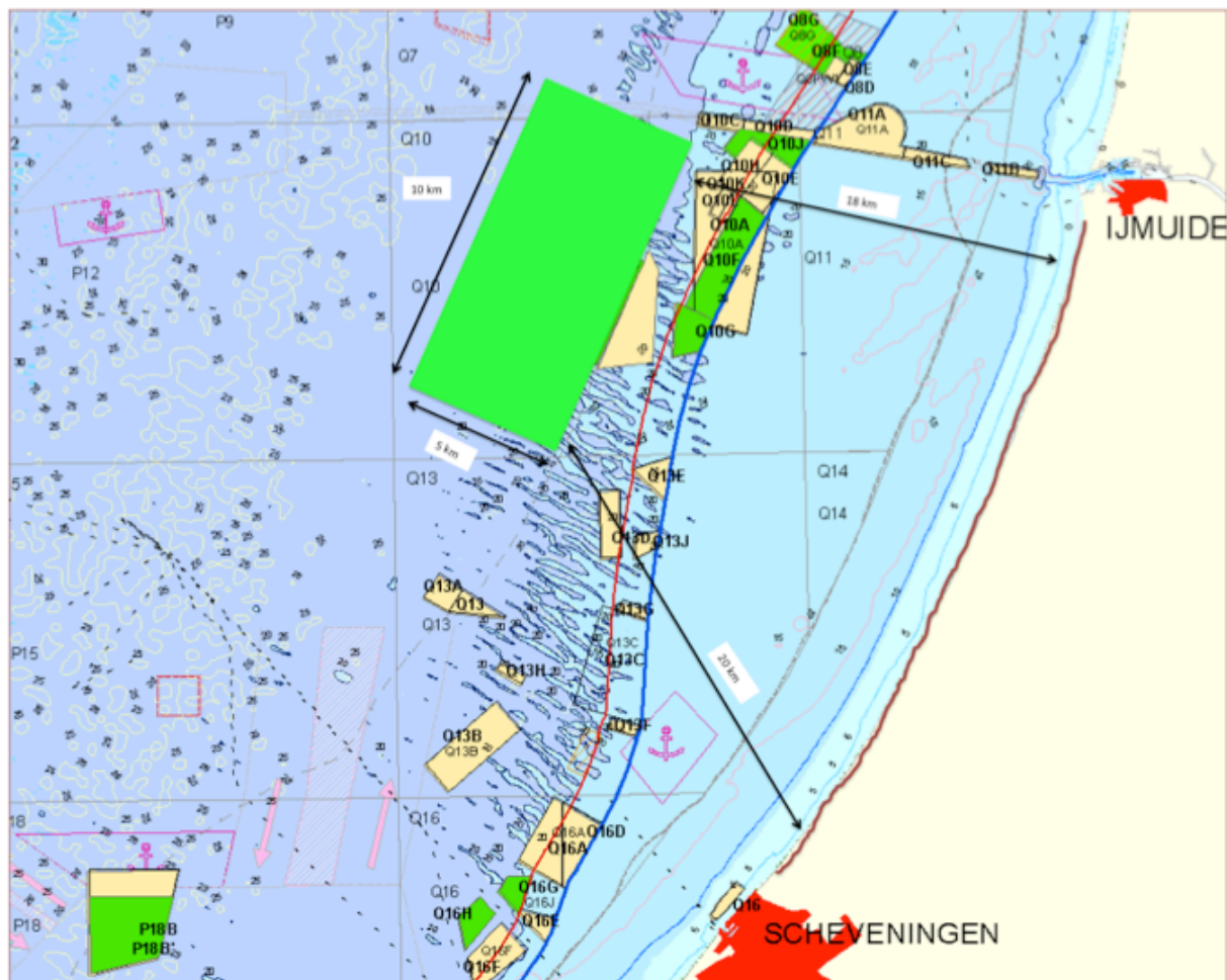
AFBEELDING 4.1 DE SITUATIE TER HOOGTE VAN NOORDWIJK.
