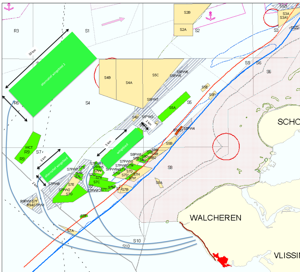
AFBEELDING 4.3 SITUATIESCHETS VAN DE ZEEUWSE BANKEN
